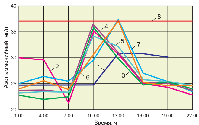
Рис. 8. Концентрация азота аммонийного в поступающей воде 2012 г.: 1 – 17 декабря; 2 – 18 декабря; 3 – 19 декабря; 4 – 20 декабря; 5 – 21 декабря; 6 – 22 декабря; 7 – 23 декабря; 8 – проектное значение (37 мг/л)
